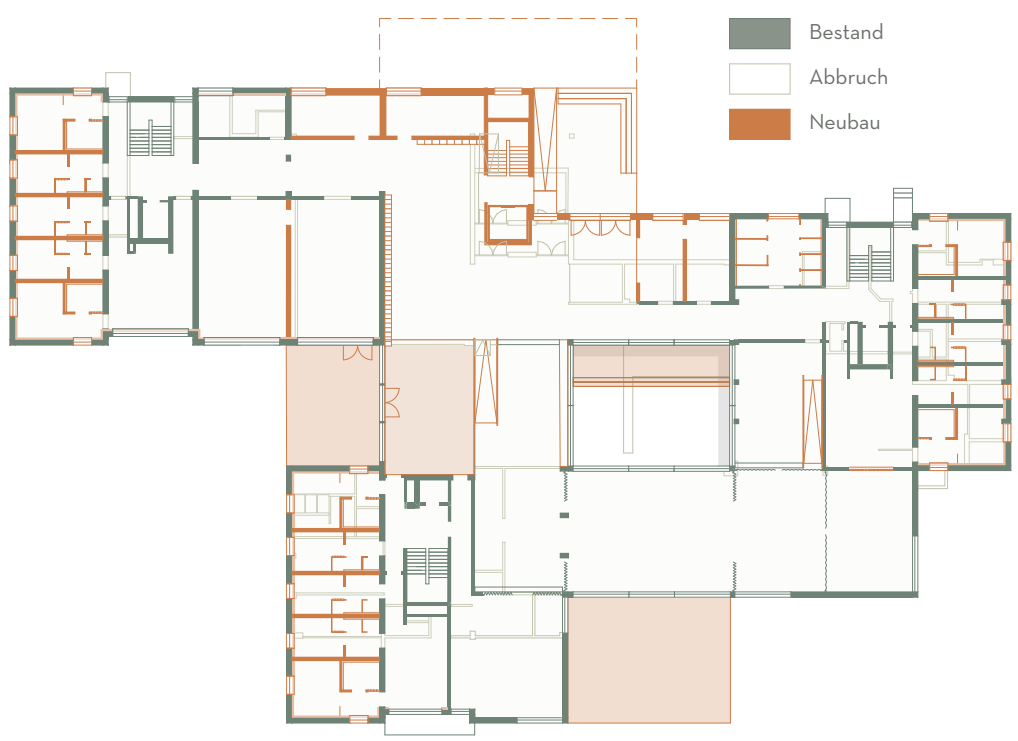
Erdgeschoss | 1:500
